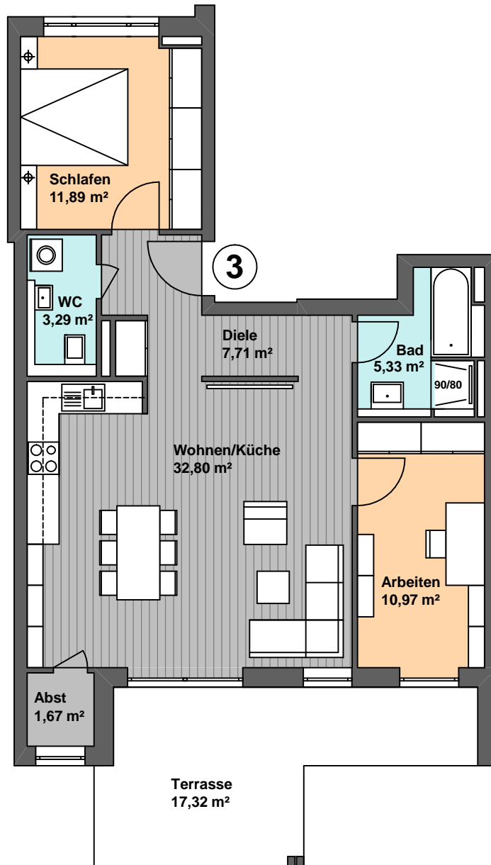
Wohnung 3 82,32m 2
