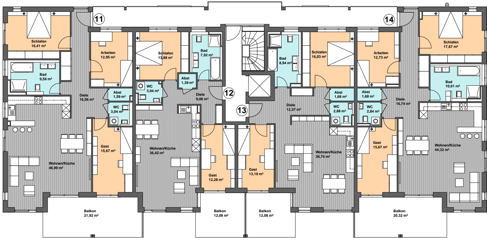
Wohnung 11 133,73m 2
